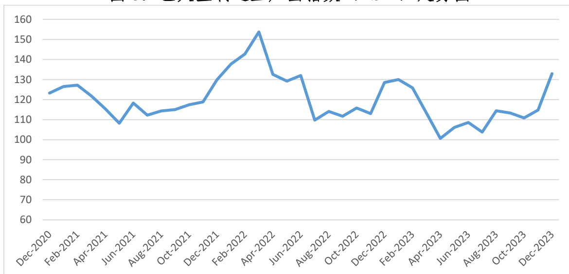
图 8：巴大型制造业产出指数（LSM）走势图
