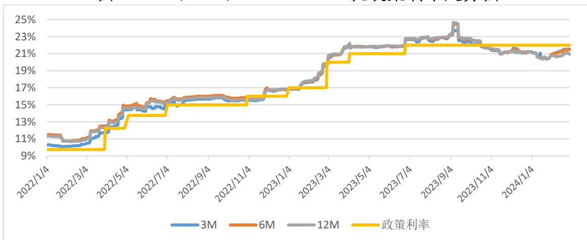
图 2：3M、6M、12M KIBOR 及政策利率走势图
