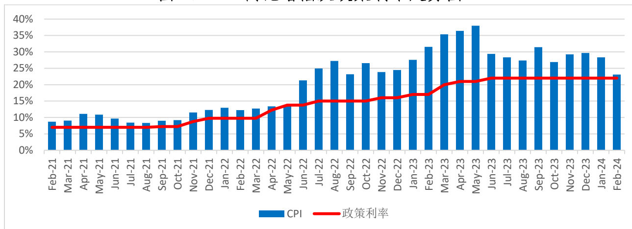
图 1：CPI 同比增幅及政策利率走势图
