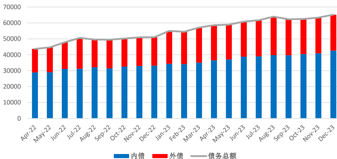
图 9：巴中央政府债务规模结构及变化趋势（十亿卢比）
